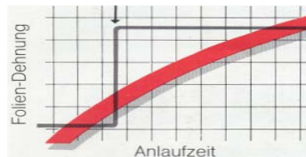
Abrißgefahr bei herkömmlichen Wickelverfahren
